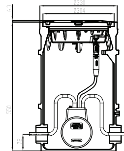
图1. 12吋深桶底座安装
