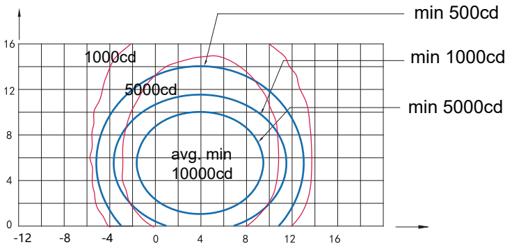
跑道入口灯（绿光），ICA0 图A2-3
