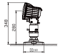
图2. 法兰盘直接安装
