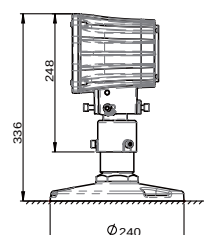
图2. 法兰盘直接安装
